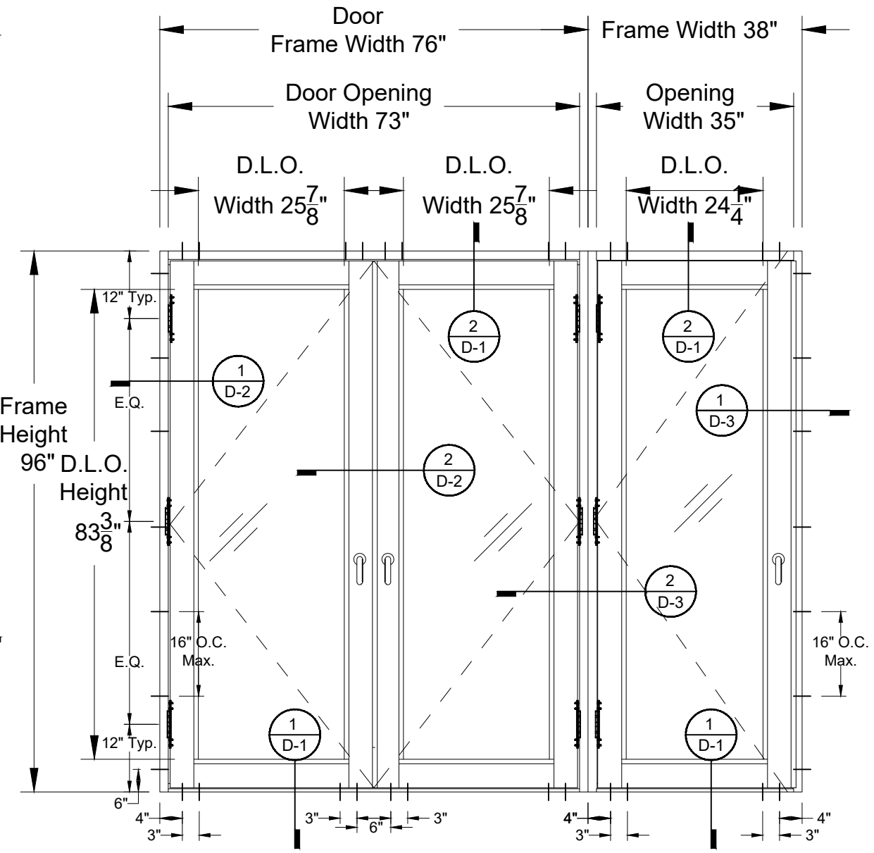
DOUBLE-SINGLE DOOR TYP. ELEVATION
