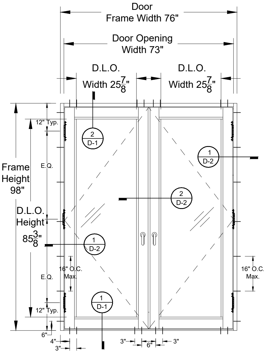
DOUBLE DOOR TYP. ELEVATION
