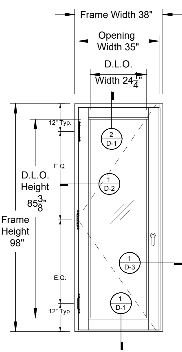
SINGLE DOOR TYP. ELEVATION
